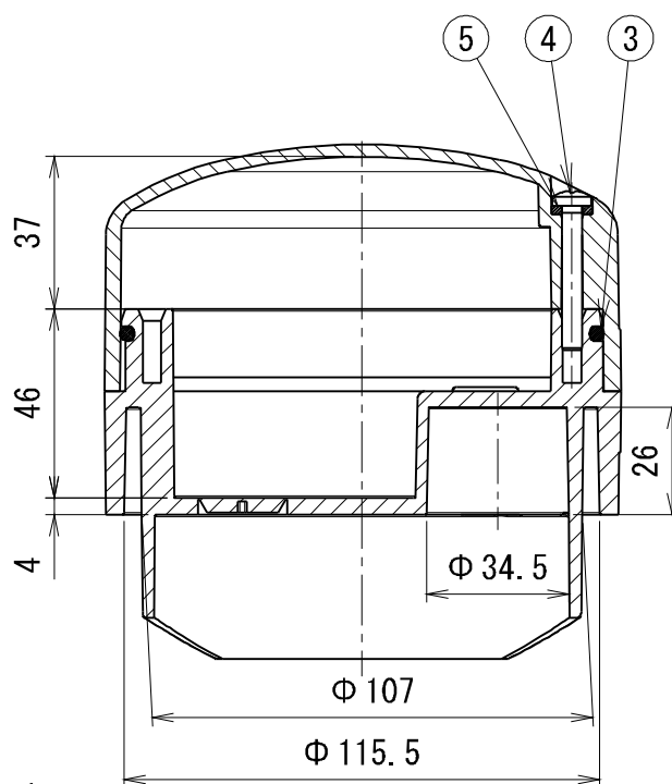
A-A断面図
